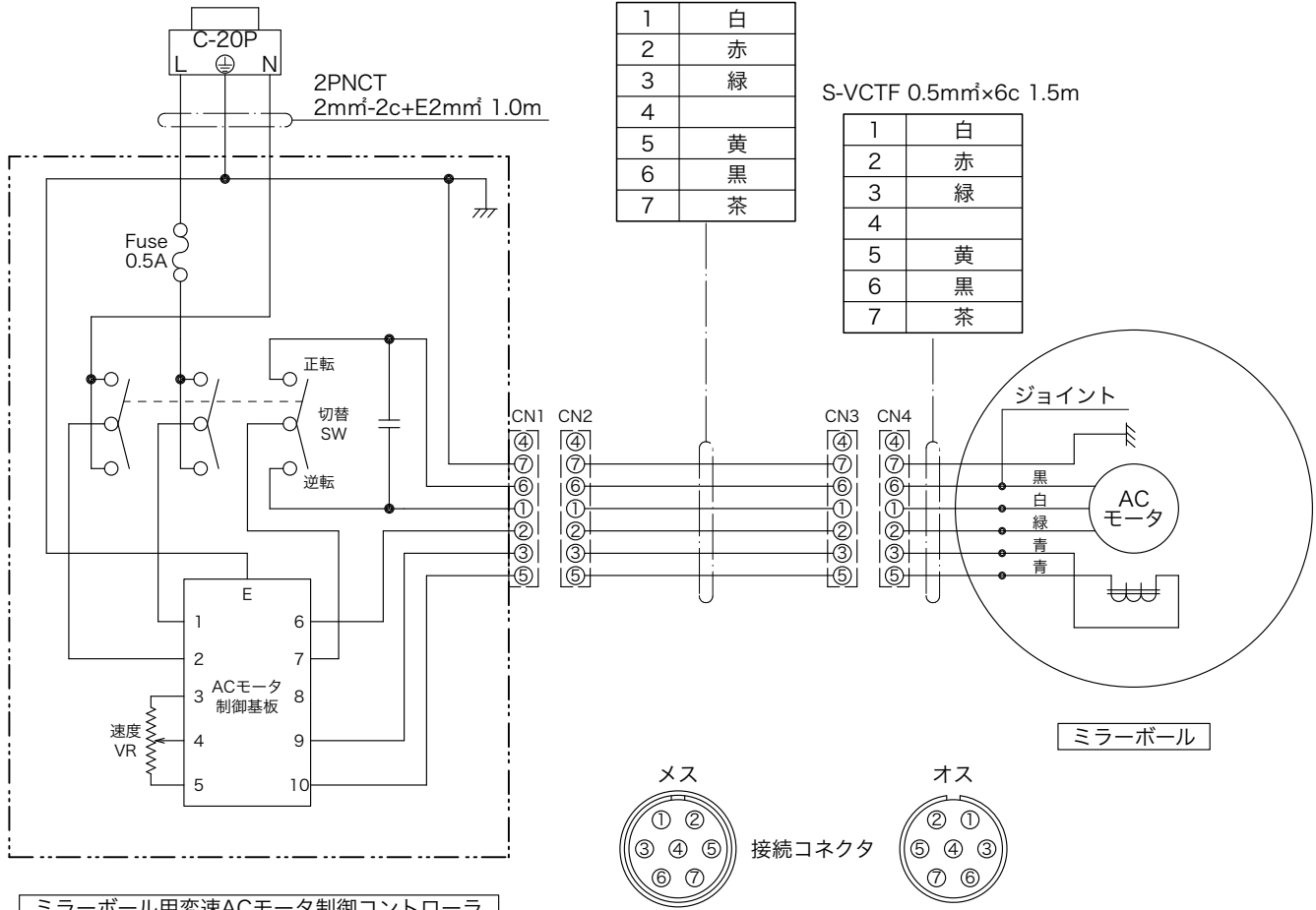
ミラーボール用変速ACモータ制御コントローラ
