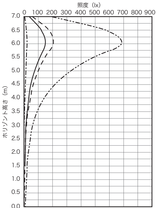
《照度曲線》・鉛直照度グラフ <照射距離:1.5m>
