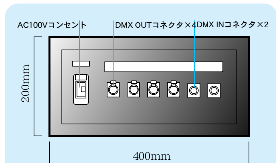
舞台袖外部信号コネクタ盤
