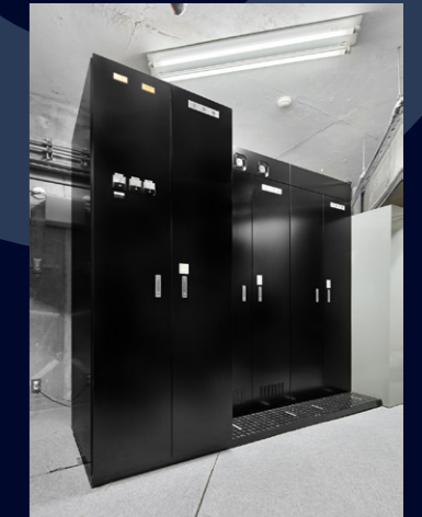
主幹盤・調光器盤・直電源盤 [交換]
